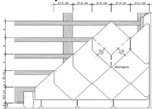
A felújítandó palafedés méretei és rögzítései
